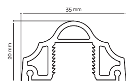
Petite Moulure 35 mm (sans possibilité de vitrer)
